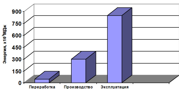
Диаграмма 1 Затраты энергии в ПЖЦ автомобиля
