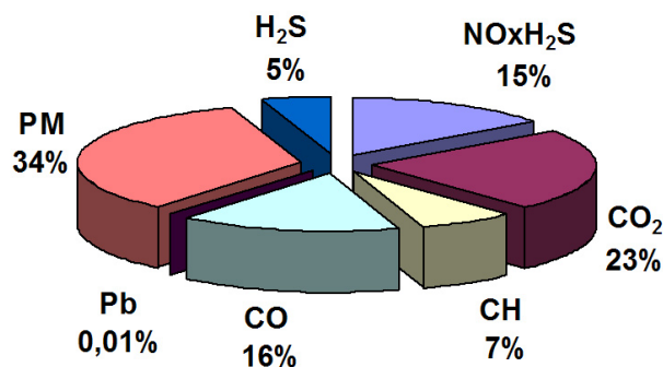
Диаграмма 2 Влияние различных веществ на загрязнение окружающей среды в ПЖЦ автомобиля
