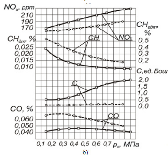
Рис. 1. Влияние применения природного газа на экологические показатели дизеля с турбонаддувом 4ЧН 11,0/12,5 в зависимости от изменения нагрузки при \Theta_{\text{впр}} = 11^\circ \text{ п.к.в.} :
