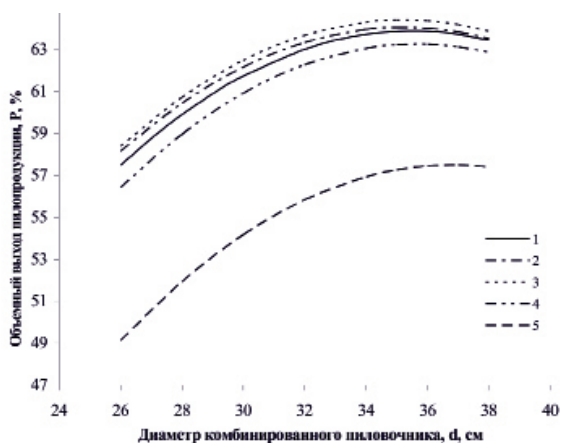
Рис. 1. Зависимость объемного выхода пилопродукции от диаметра комбинированного пиловочника для различных вариантов удаления коры и гнили ( d_r = 18 см, l = 6 м)
