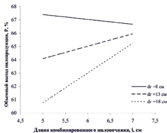
Рис. 3. Зависимость объемного выхода пилопродукции из комбинированного пиловочника от его длины при различных диаметрах гнили
