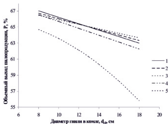
Рис. 4. Зависимость объемного выхода пилопродукции из комбинированного пиловочника от диаметра гнили в комлевом торце при удалении коры и гнили различными способами ( d = 32 см, l = 6 м)
