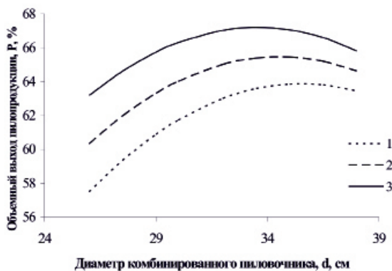
Рис. 2. Зависимость объемного выхода пилопродукции от диаметра комбинированного пиловочника для варианта удаления коры и гнили перпендикулярно пластям ( l = 6 м): 1 – d_r = 18 см; 2 – d_r = 3 см; 3 – d_r = 8 см
